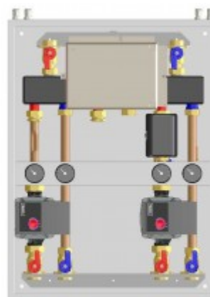
MODUŁ WIELOSTREFOWY - SIM 2Z typ 1LTE.1HT.YP
