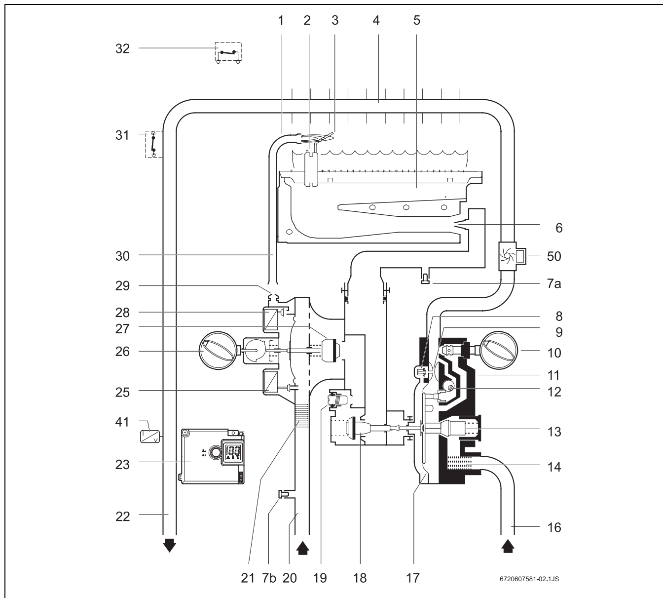
Rys. 2 Schemat działania
