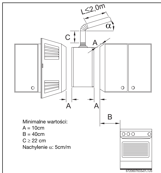
Rys. 4 Minimalne odległości
