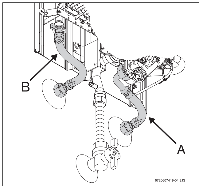
Rys. 5 Podłączanie wody
