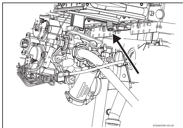
Rys. 14 Punkt pomiaru ciśnienia
