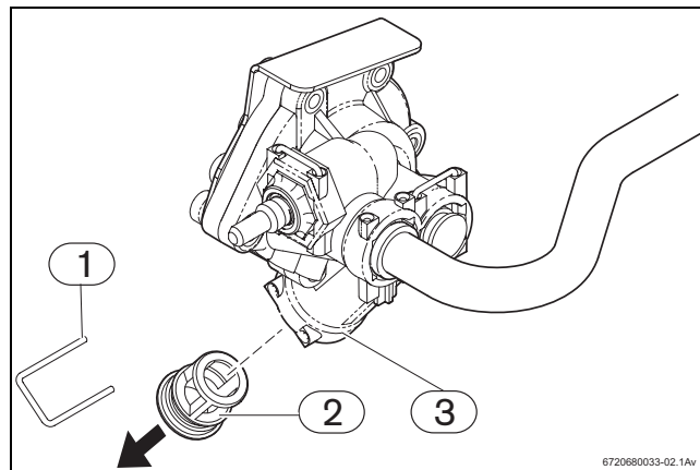
Rys. 13 Opróżnianie ogrzewacza
