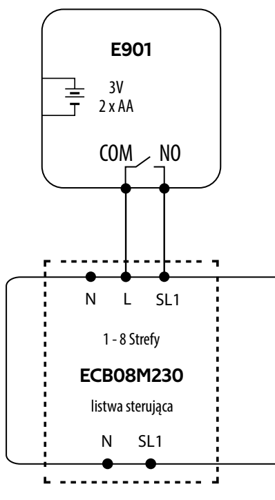
c) Schemat podłączenia do listwy sterującej
