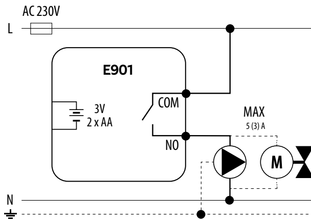
b) Schemat podłączenia do pompy / siłownika
