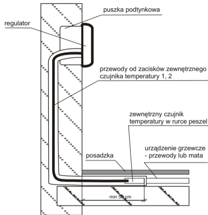
Rys. I - Zalecany sposób montażu czujnika temperatury
